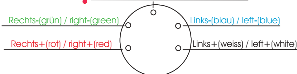
Lötseitige Ansicht / solderside view
